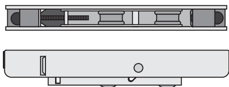
ROLDANA DUPLA COM BALANCIM LINHA130 Cód.: YD808
