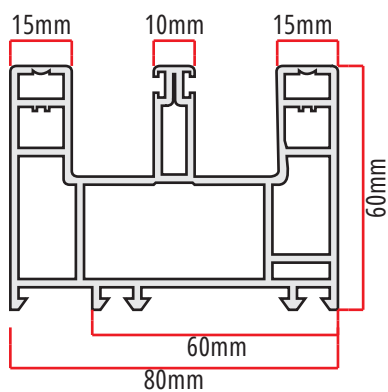
MC-130 1696gr/m marco de correr extra-pesado MAXXI
