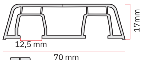
ARREMATE 0 (com click) 0,455gr/m
