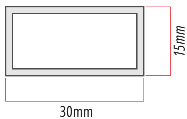
TUBO 30X15 0,195 gr/m
