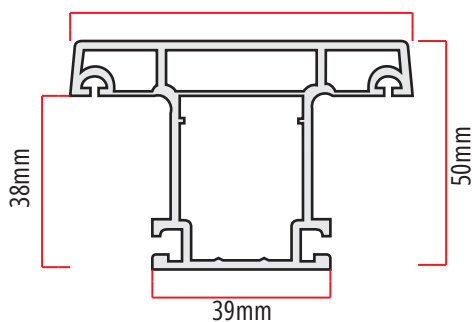
TC-130 1096gr/m travessa para folha de correr extra-pesada MAXXI 75mm
