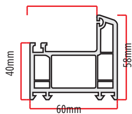
MA-60 1094gr/m marco fixo, abrir, maximar e oscilobatente médio e pesado euroTEC | TECplus
