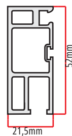
BT-37 197gr/m batedor para folha de tela leve iTEC | euroTEC
