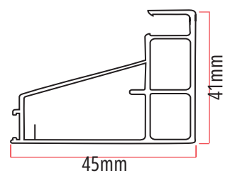
FMA - 45 507gr/m folha mosquiteiro abrir euroTEC | TECplus MAXXI
