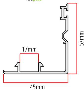
MAO-100 419gr/m mão de amigo para folha de correr pesada TECplus
