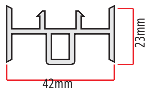
B-37 309gr/m batedor para folha de correr leve e média iTEC | euroTEC
