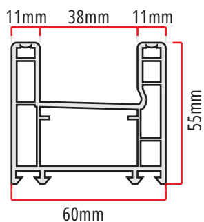
MC-60-2T 915gr/m marco padrão de correr 2 trilhos iTEC euroTEC TECplus
