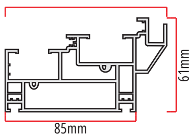
MG-85 1664gr/m marco guilhotina automático leve euroTEC
