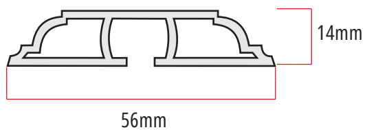
ARREIMATE DECORATIVO 314gr/m
