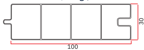
PALHETA PAINEL100 NOVA 0,643gr/m
