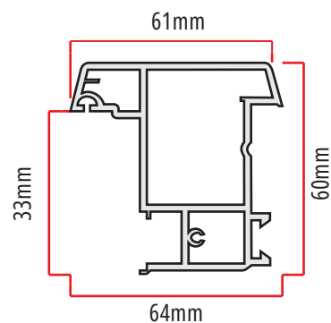
TFS-60 980gr/m travessa falsa do sistema de abrir euroTEC | TECplus
