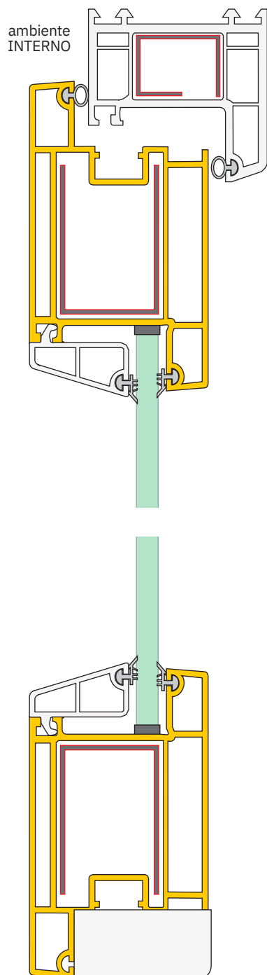
Porta de abrir (para dentro) sem marco inferior TECplus-100
