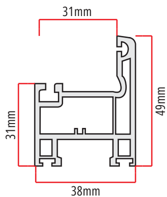
FG-85 681gr/m folha guilhotina automática leve euroTEC
