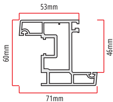
FAD-60 1123gr/m folha oscilobatente e abrir (para dentro) média euroTEC
