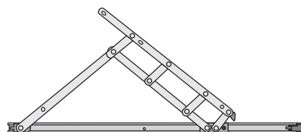
BRAÇO EM INOX 24" espessura: 15mm Cód.: H2482016
