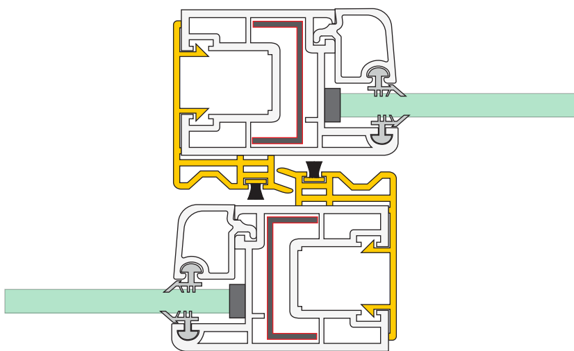
Mão de amigo euroTEC
