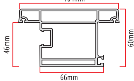
FAF-60plus 1568gr/m folha oscilobatente e abrir (para fora) pesada TECplus 104mm
