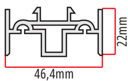
B-42 388gr/m batedor para folha de correr pesada TECplus
