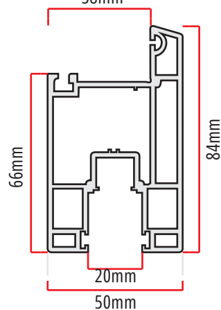
FC-130 1467gr/m folha de correr extra-pesada MAXXI 38mm
