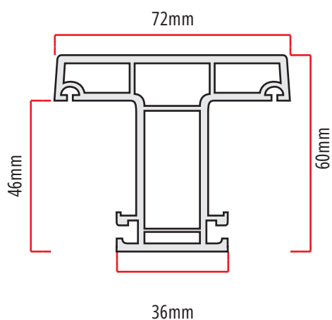
TA-60 1193gr/m folha maximar média travessa do sistema de abrir euroTEC | TECplus
