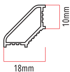
ARREMATE 2 (externo) 80gr/m
