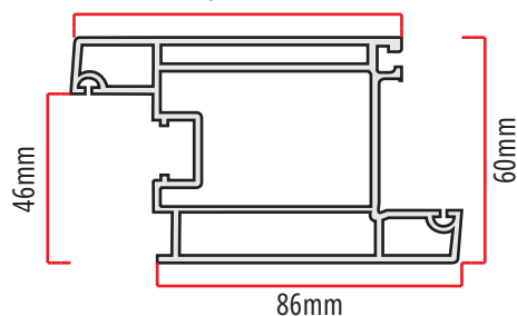
FAD-60plus 1568gr/m folha maximar e abrir (para dentro) pesada TECplus 84mm
