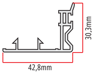
MAO-55 278gr/m mão de amigo para folha de correr leve iTEC
