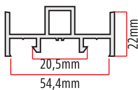
B-50 415gr/m batedor para folha de correr extra-pesada MAXXI
