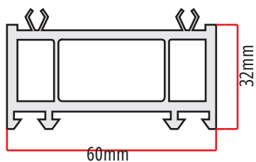
PM-60 828gr/m prolongador de marco de 60mm iTEC | euroTEC | TECplus
