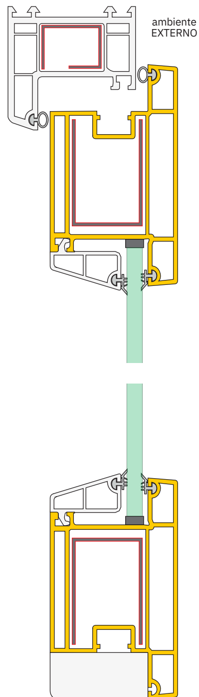
Porta de abrir (para fora) sem marco inferior TECplus-100
