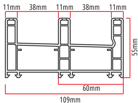
MC-60-3T 1415gr/m marco padrão de correr 3 trilhos iTEC euroTEC TECplus
