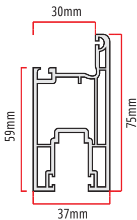
FC-75 920gr/m folha de correr média euroTEC
