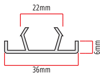
T-85 168gr/m tampa do marco guilhotina leve euroTEC
