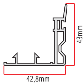
MAO-75 295gr/m mão de amigo para folha de correr média euroTEC
