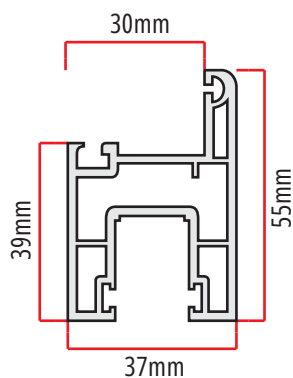
FC-55 695gr/m folha de correr leve marco de maximar leve iTEC
