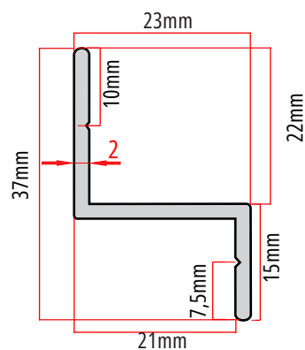
ESPAÇADOR DE PISO 0,178 gr/m
