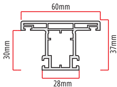
TC-55 635gr/m travessa de de correr leve e média folha de maximar leve iTEC
