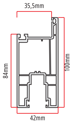
FC-100 1370gr/m folha de correr pesada TECplus
