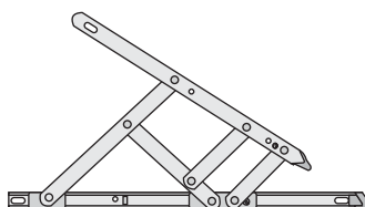
BRAÇO EM INOX 16" Cód.: H1682016
