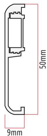
ARREMATE 1 (com tampa) 210gr/m
