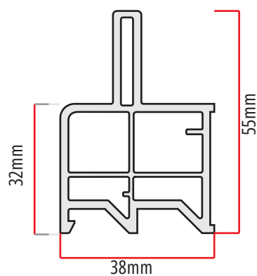
MCT-60 566gr/ marco adicional para tela mosquito leve iTEC | euroTEC
