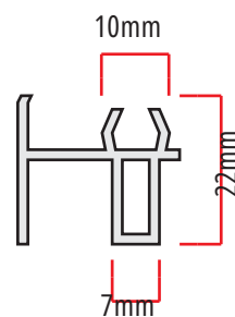
BT-37 197gr/m batedor para folha de tela leve iTEC | euroTEC
